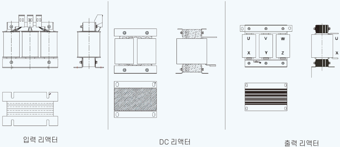
출력 리액터
